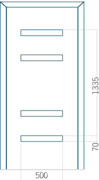
Technický výkres
