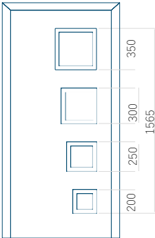
Technický výkres
