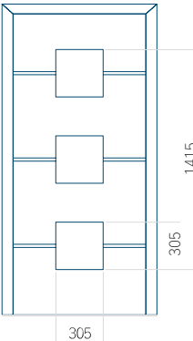
Technický výkres
