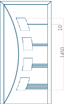
Technický výkres
