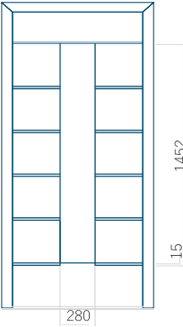
Technický výkres
